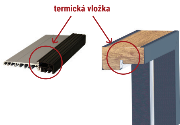
Prierez termickej hliníkovo-drevenej zárubne
