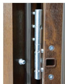
3D pánty nastaviteľné v 3 rovinách
