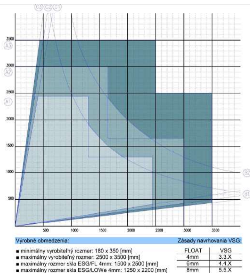
Graf 1 Doporučené hrúbky skiel v závislosti na rozmeroch a ploche – DVOSKLO
